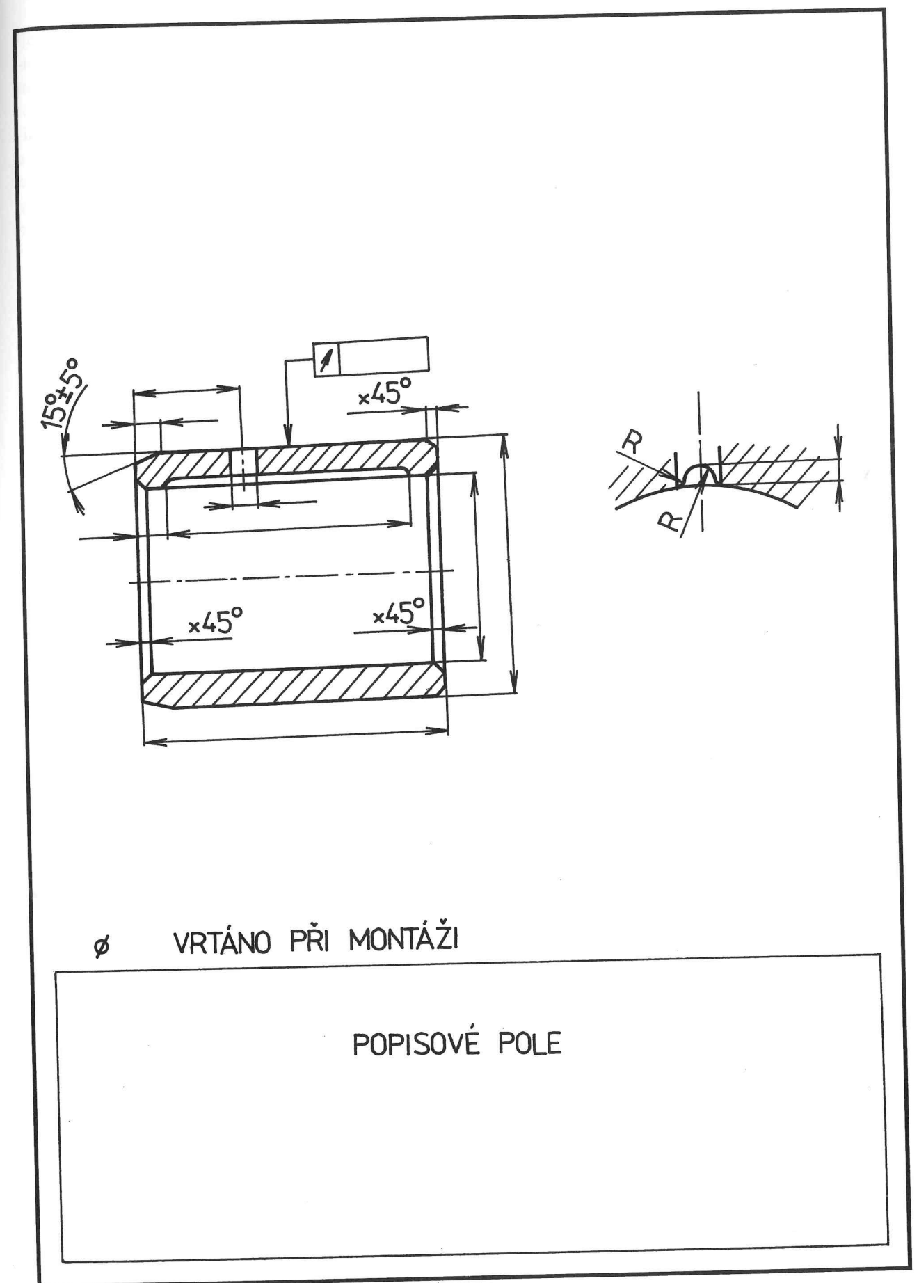
Obr. 285 Předtisk výrobního výkresu pro opakující se výrobu
