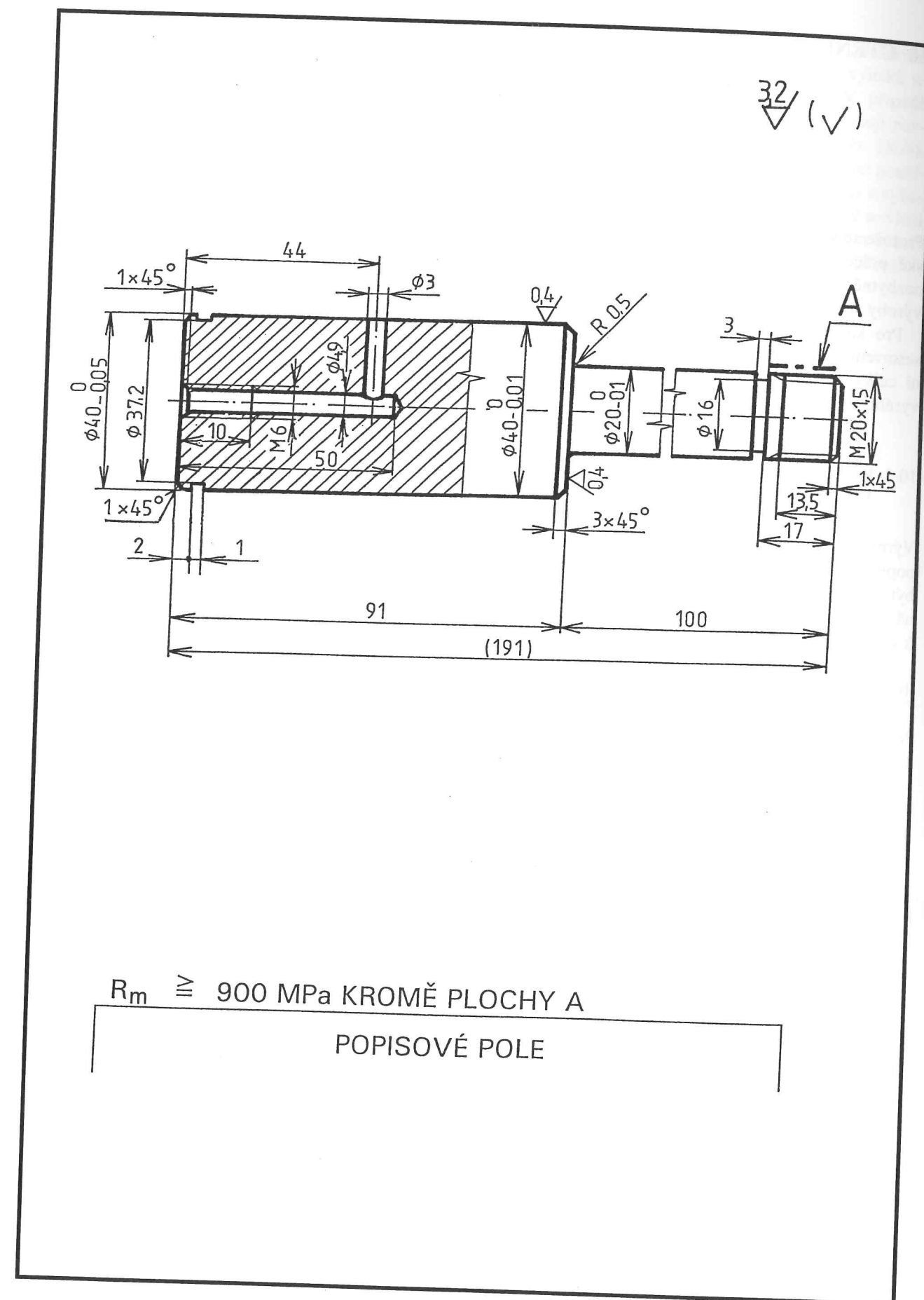
Obr. 284 Výrobní výkres součásti
